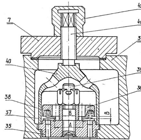
Рис.13. Клапан нагнетательный I ступени
