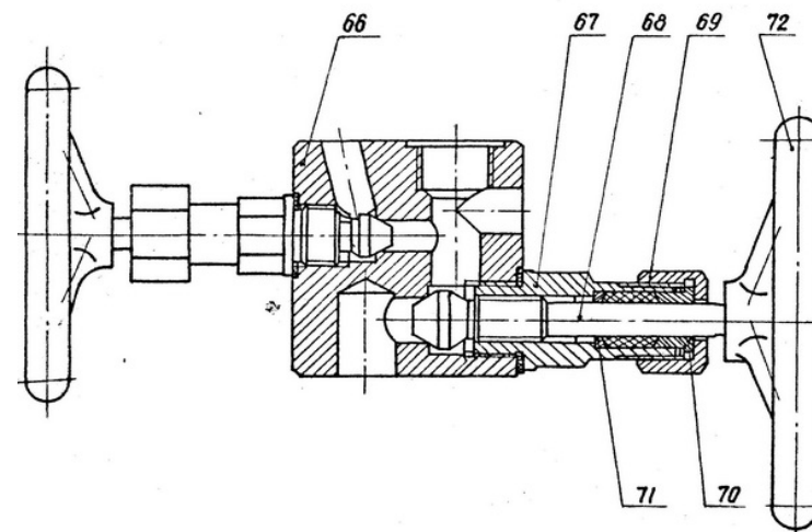
Рис.18. Вентиль запорный и продувочный
