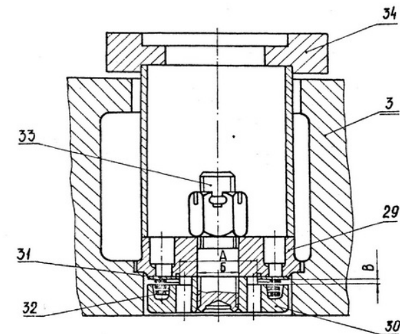
Рис.12. Клапан всасывающий I ступени
