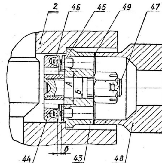
Рис.14. Клапан всасывающий II ступени
