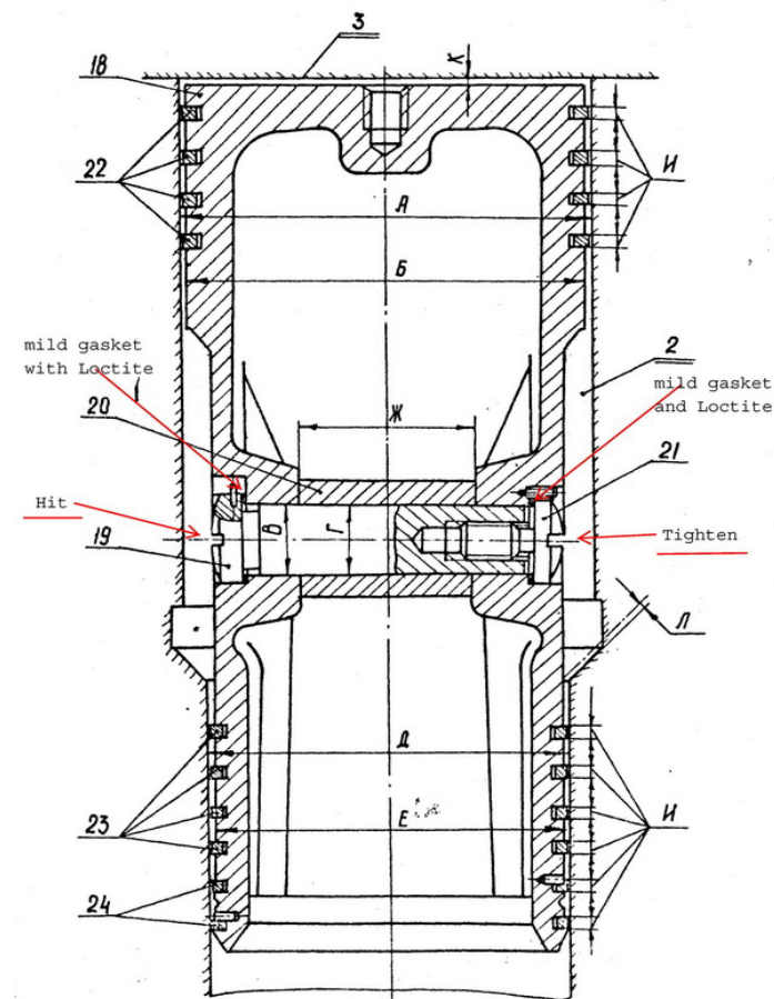
Рис. 10. Поршень
