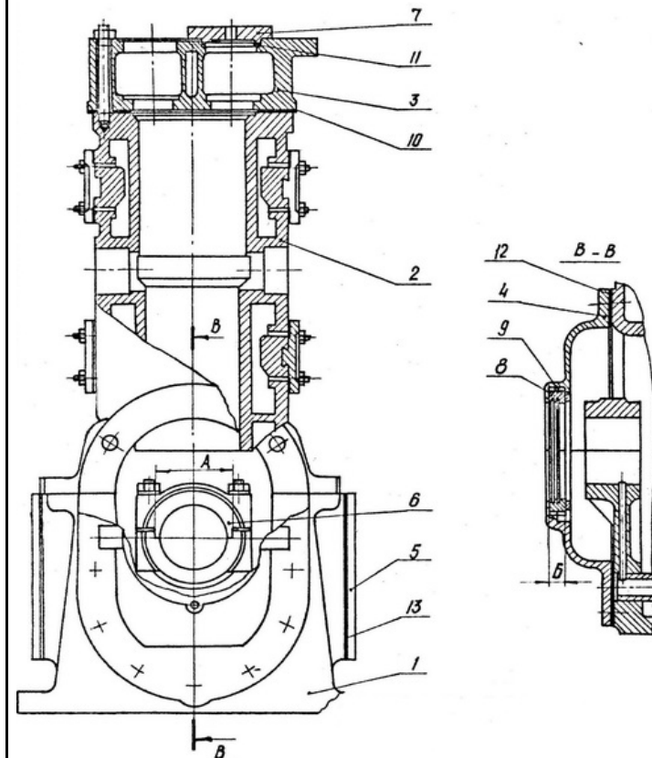
Рис.6. Картер и цилиндры
