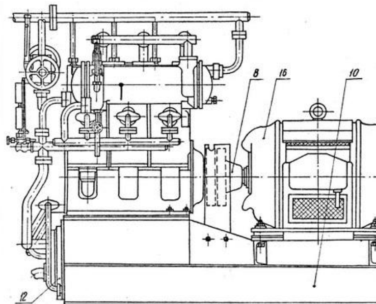
Рис. I. Компрессоры типа ЭКП
