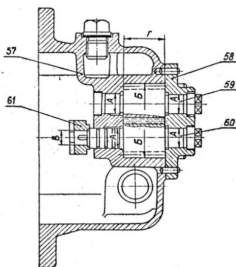
Рис.16. Насос масляный
