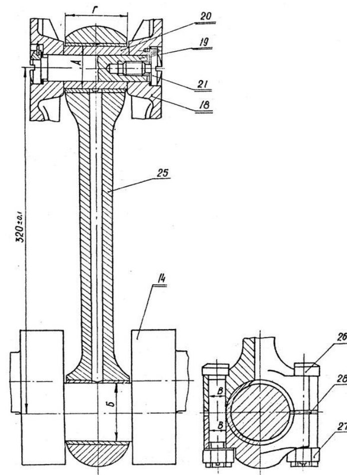
Рис. II. Шатун
