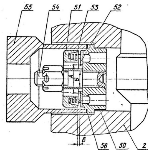
Рис.15. Клапан нагнетательный II ступени
