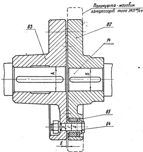
Рис.17. Муфта
